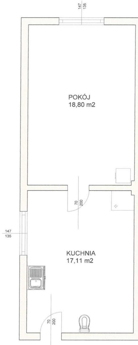
Rzut Lokalu
